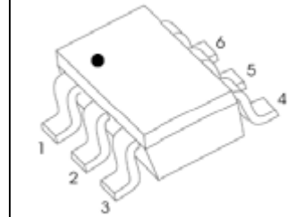
SOT-363
