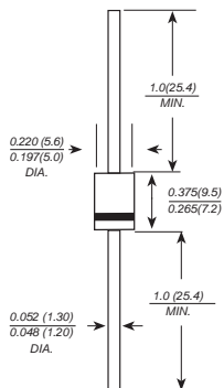
DO-201AD
