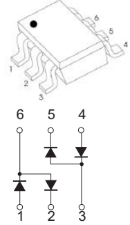
SOT-363
