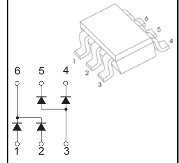
SOT-363
