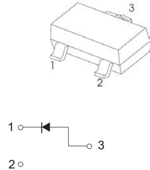
SOT-23
