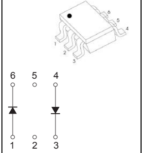
SOT-363
