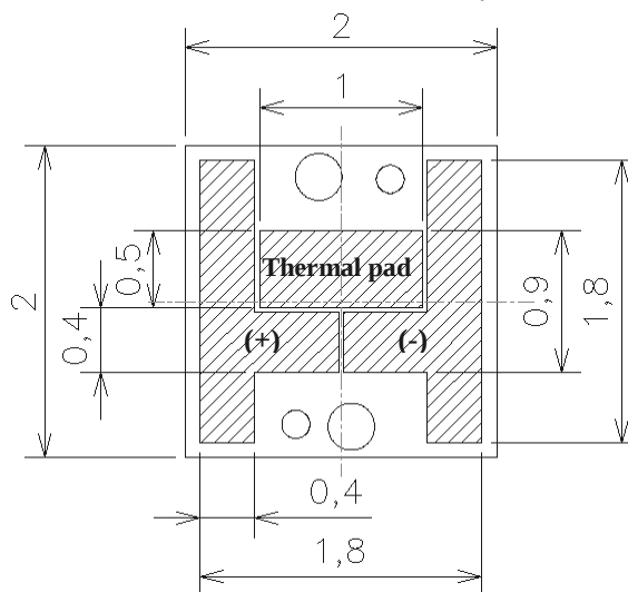
Cu pattern
