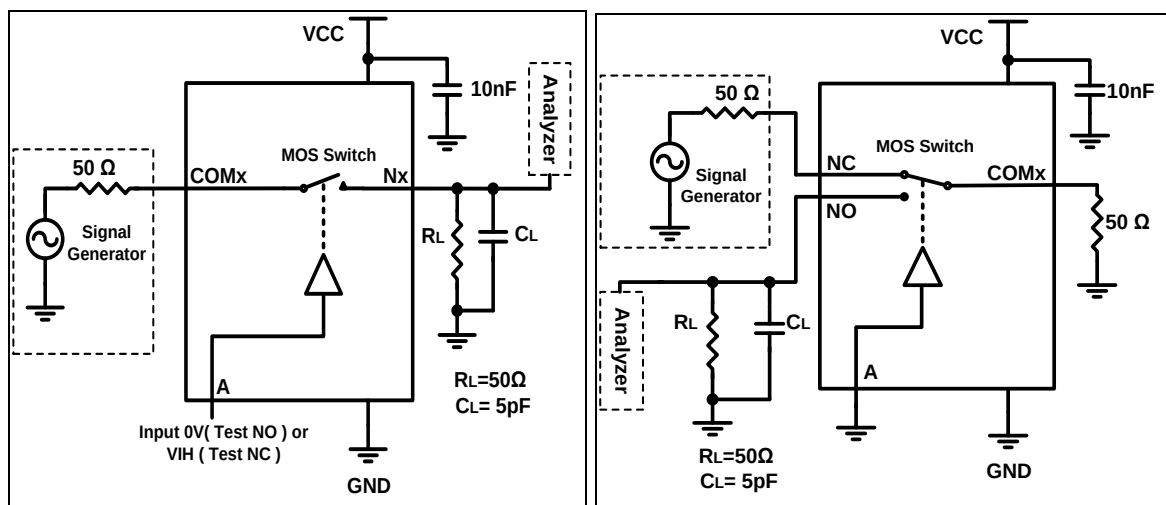
Figure4. Off Isolation ( V_{ISO} )
