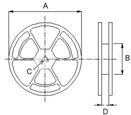
Reel Dimensions
