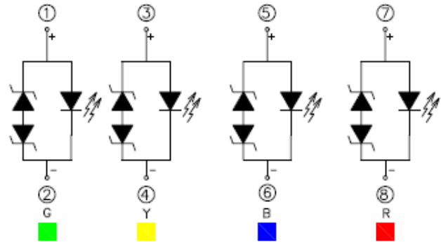
Polarity
