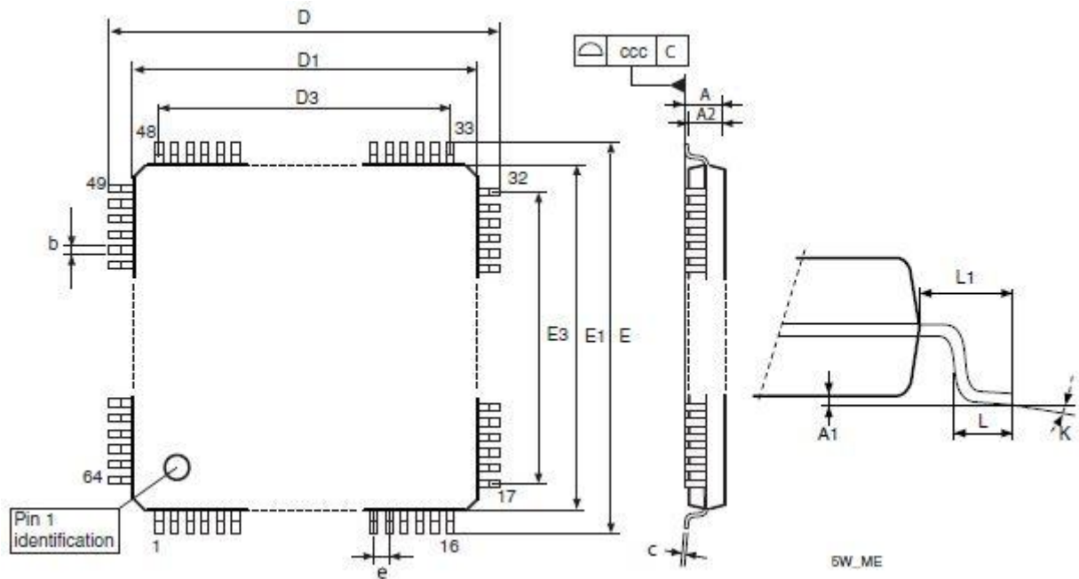
图 25 LQFP48-10x10mm, 64 脚低剖面方形扁平封装图
