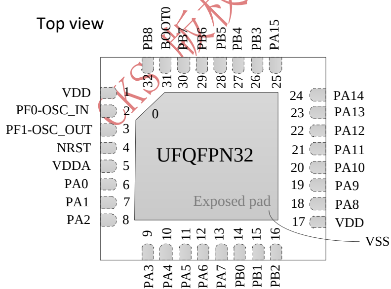
图 5 UFQFPN32 引脚封装脚位图
