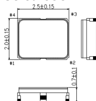
SG-8018CG
