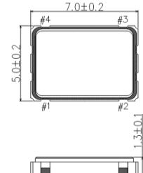
SG-8018CA
