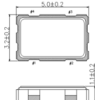
SG-8018CB
