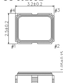
SG-8018CE
