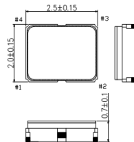
SG-8018CG
