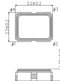
SG-8018CE
