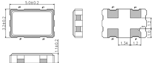
SG-9101CB
