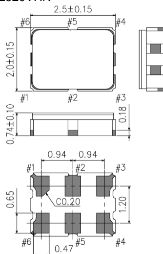
SG2520VHN
