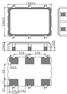
SG7050VEN
