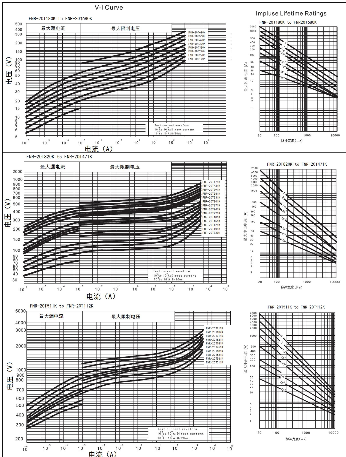
*20T 系列 V-I 特性曲线和最大浪涌电流降额曲线
