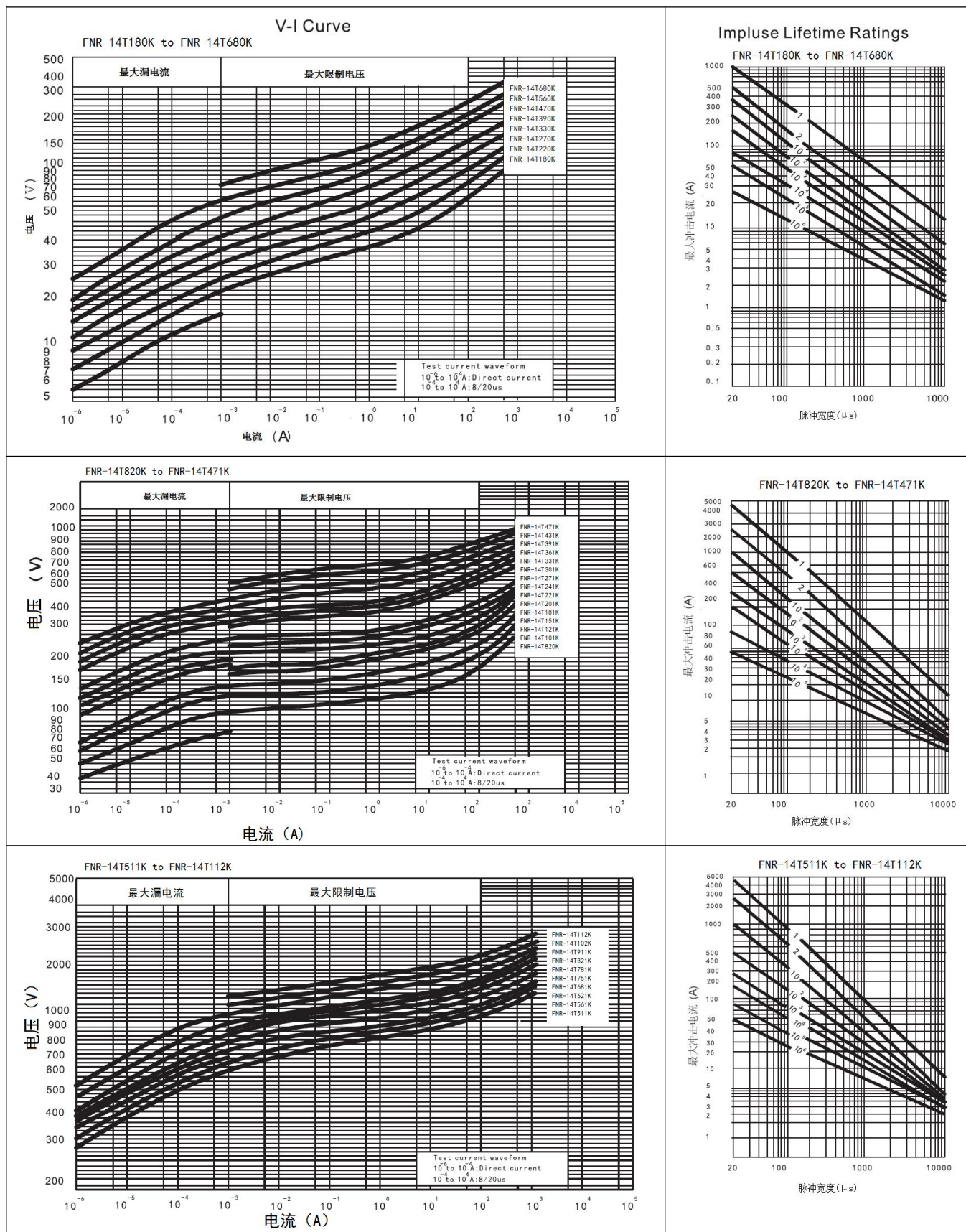
*14T 系列 V-I 特性曲线和最大浪涌电流降额曲线
