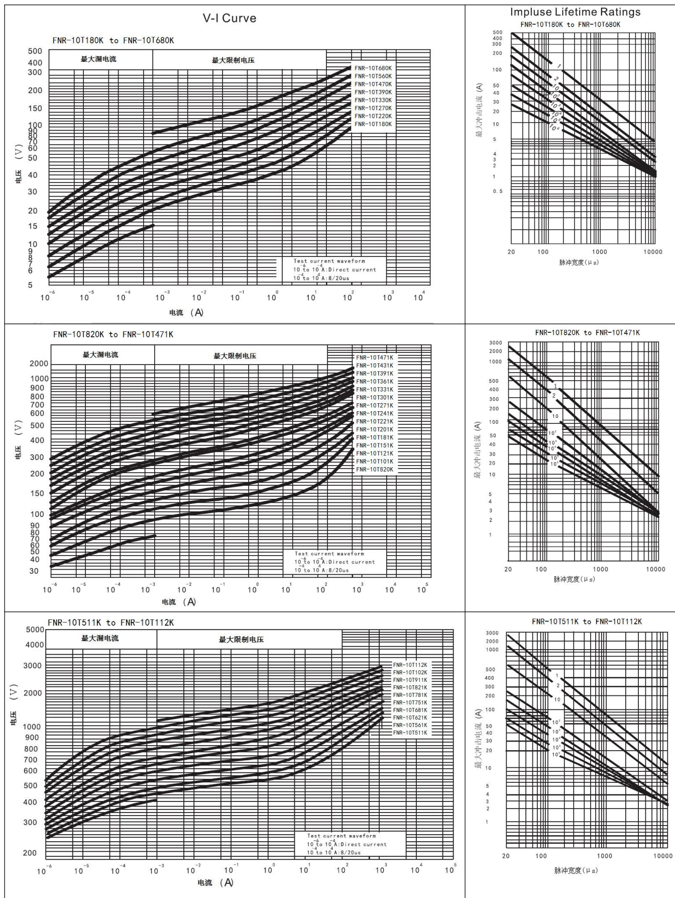
*10T 系列 V-I 特性曲线和最大浪涌电流降额曲线
