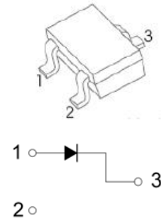
SOT-323
