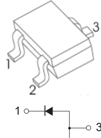
SOT-323
